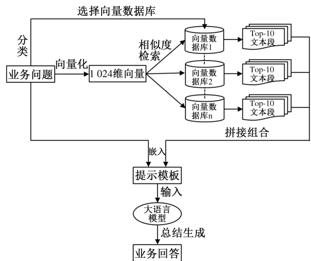
图 4 RAG 系统流程
