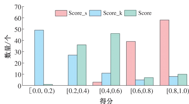
图 7 模型 T 得分频数分布
