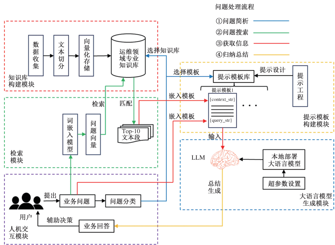
图 1 系统总体框架图 Fig. 1 Overall system framework diagram
