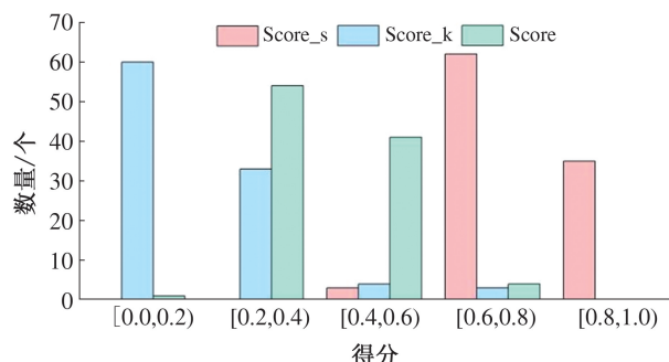
图 6 模型 Z 得分频数分布
