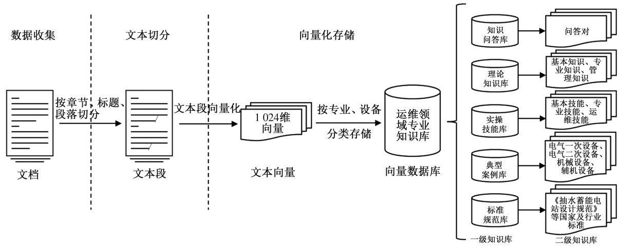
图 2 知识库构建流程 Fig. 2 Knowledge base construction process
